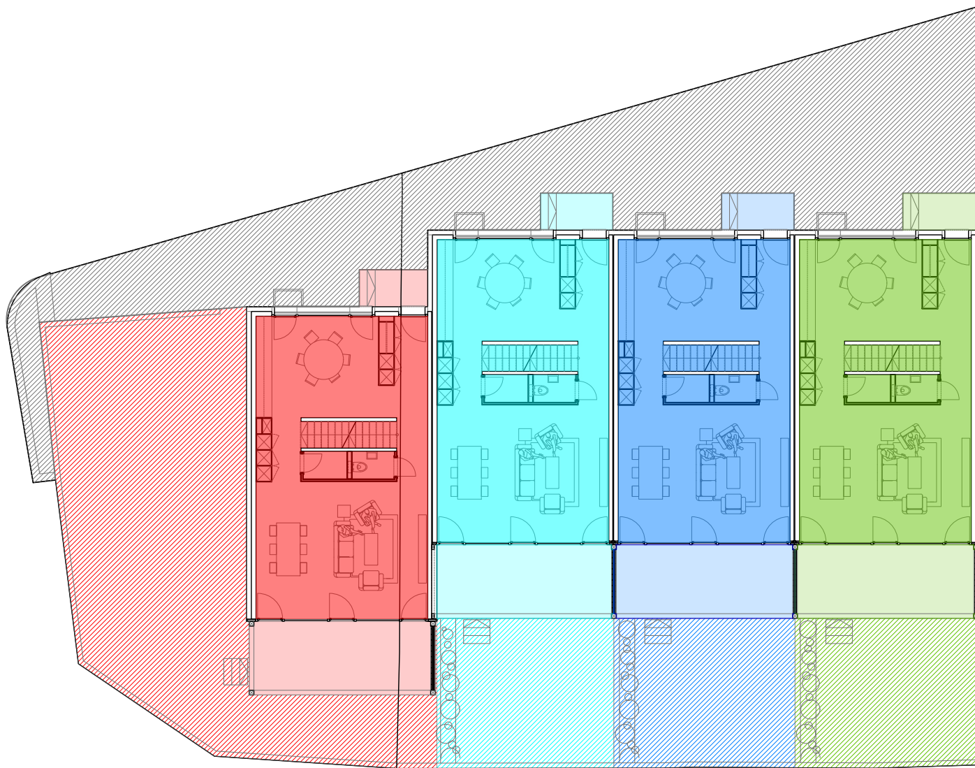
Rez-de-chaussée
